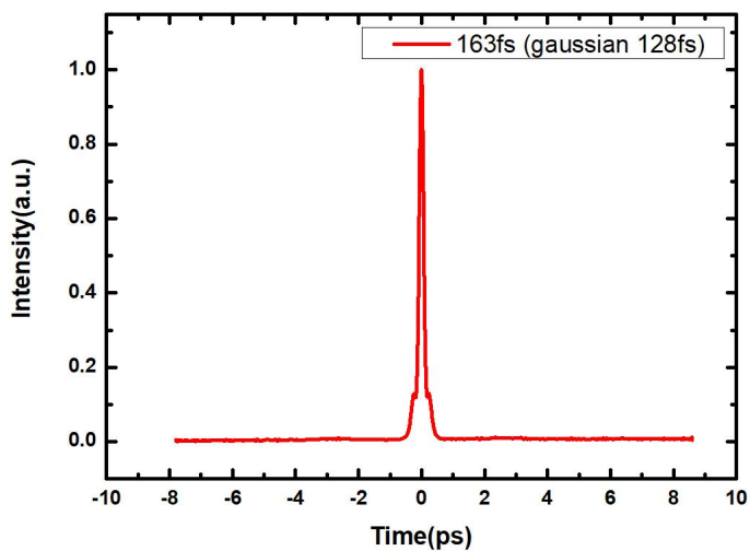
脉冲 AC 曲线
